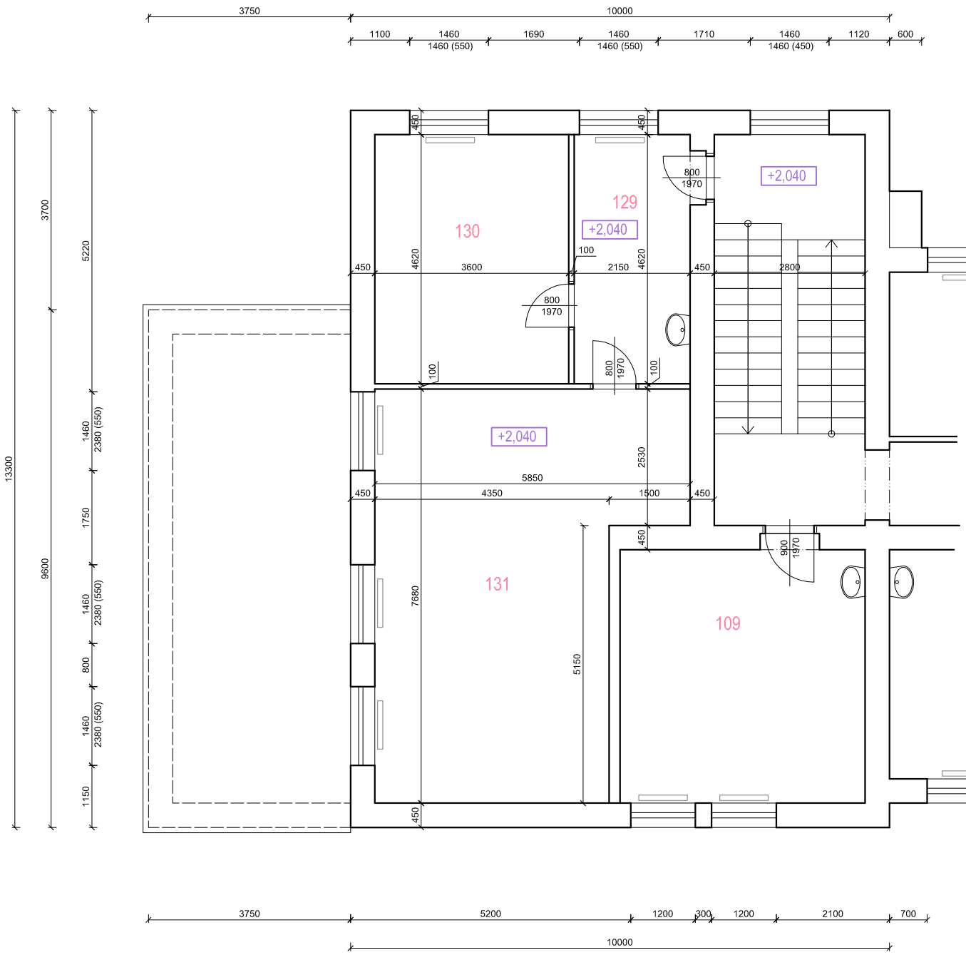
PŮDORYS MÍSTNOSTI MEZI 1.NP A 2.NP
