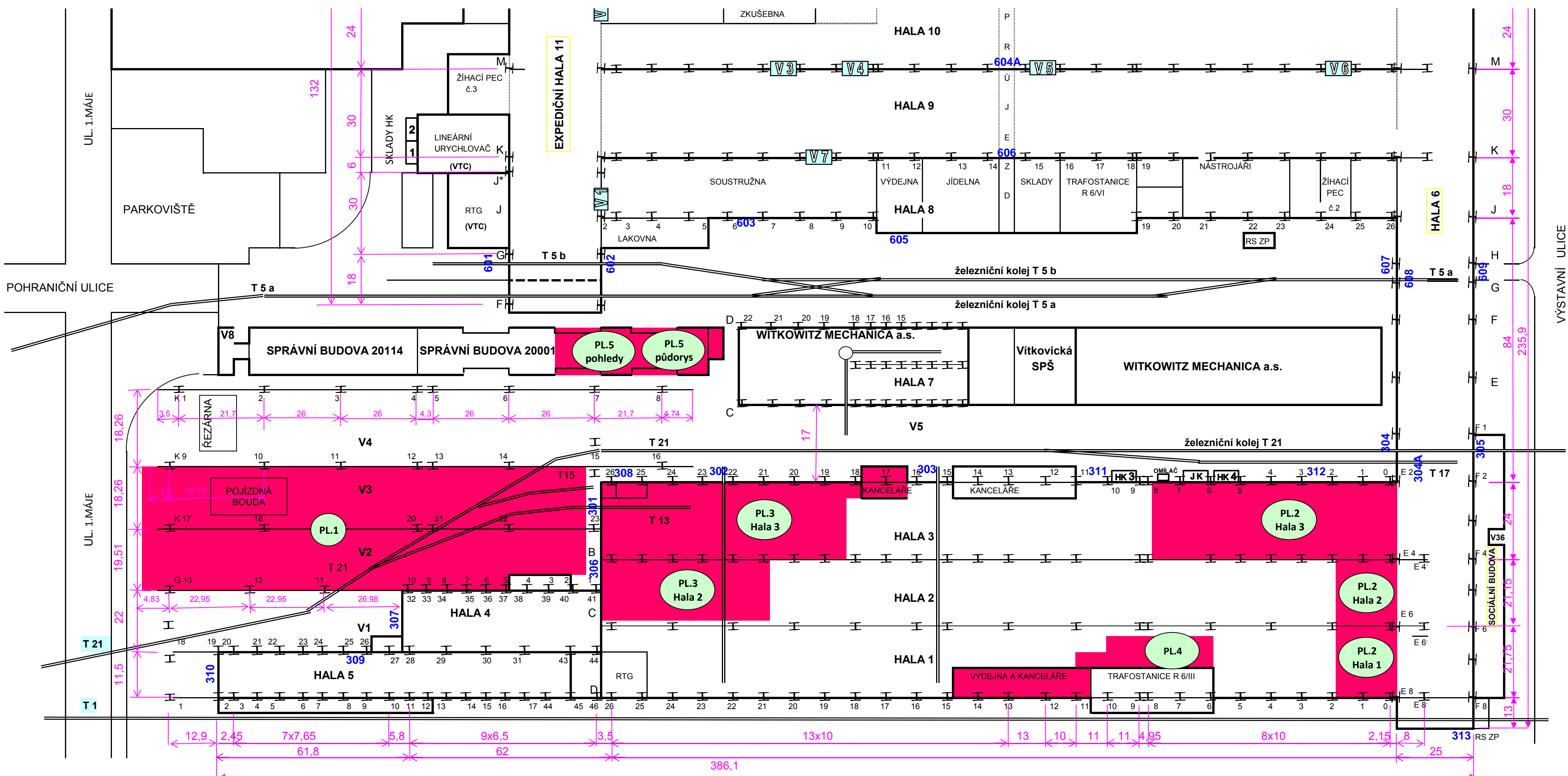
SCHÉMA a.s. VÍTKOVICE ENERGETICKÉ STROJÍRENSTVÍ Kreslil: Jiří Orzel Datum: 6/2020
